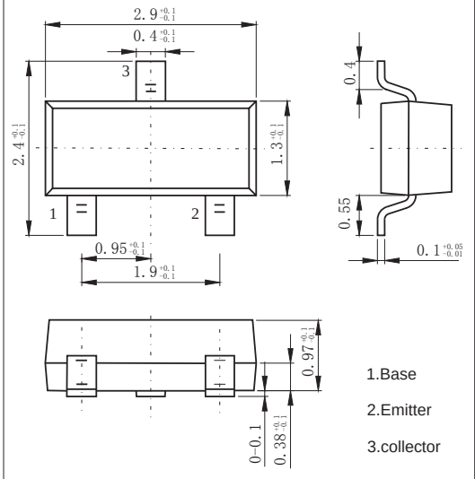
SOT-23
