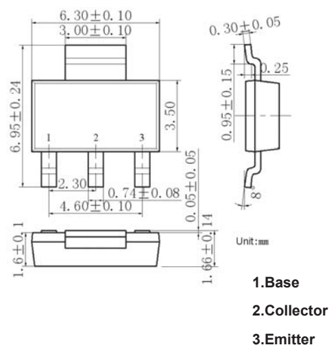
SOT-223
