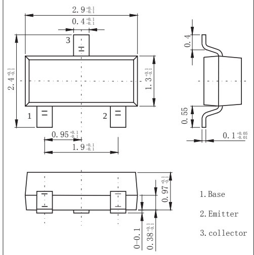
SOT-23
